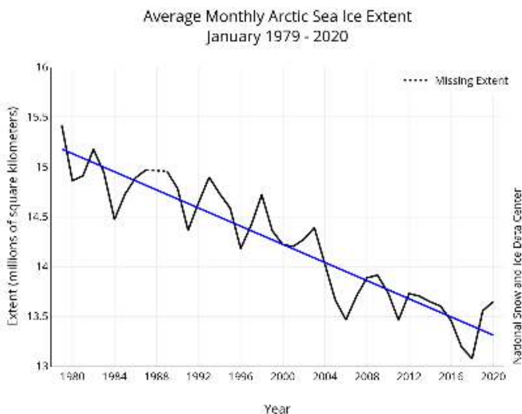
Figura 2: Serie temporale dell'estensione media del ghiaccio marino artico 7
